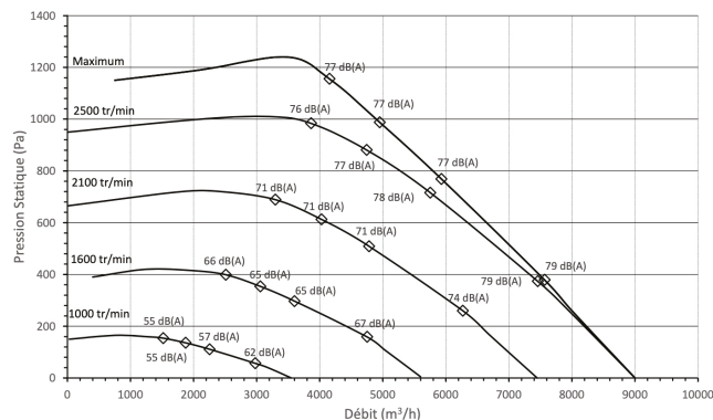
CESA 800 - (8000 m 3 /h - 2,27 kW - 10 A)
