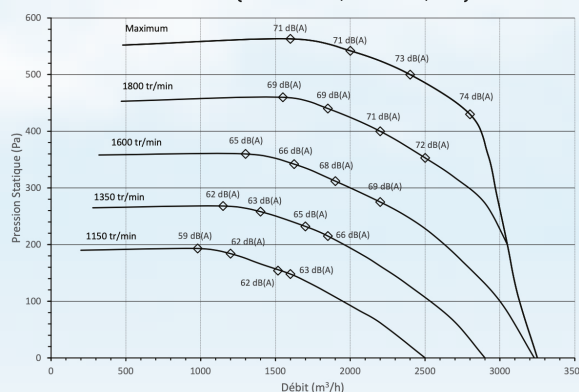
CESA 300 - (3000 m 3 /h - 1,074 kW - 4,62 A)
