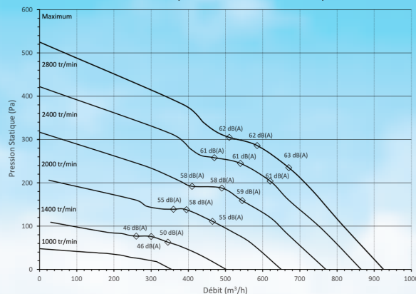
CESA 100 - (650 m 3 /h - 0,18 kW - 1,26 A)
